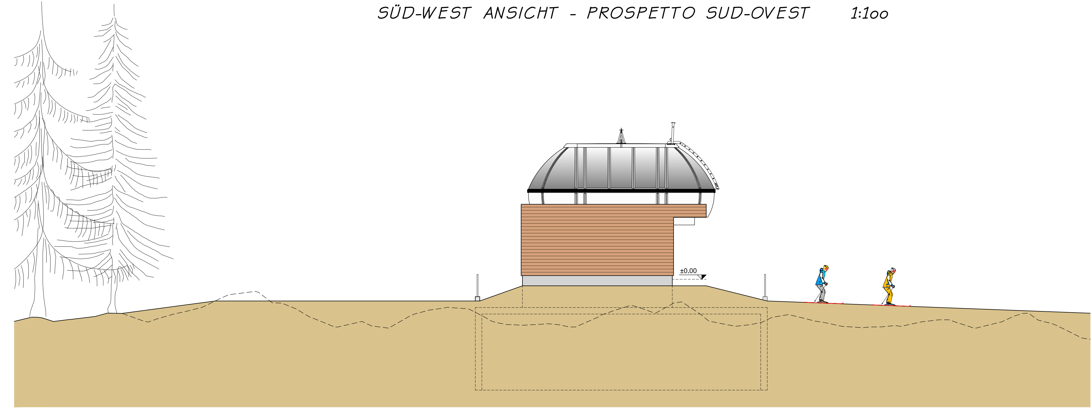
SÜD-WEST ANSICHT - PROSPETTO SUD-OVEST 1:100
