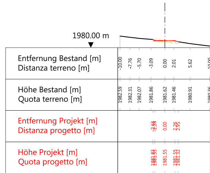
Querprofil L7 Profilo trasversale L7
