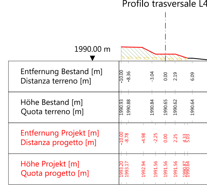
Querprofil L4 Profilo trasversale L4
