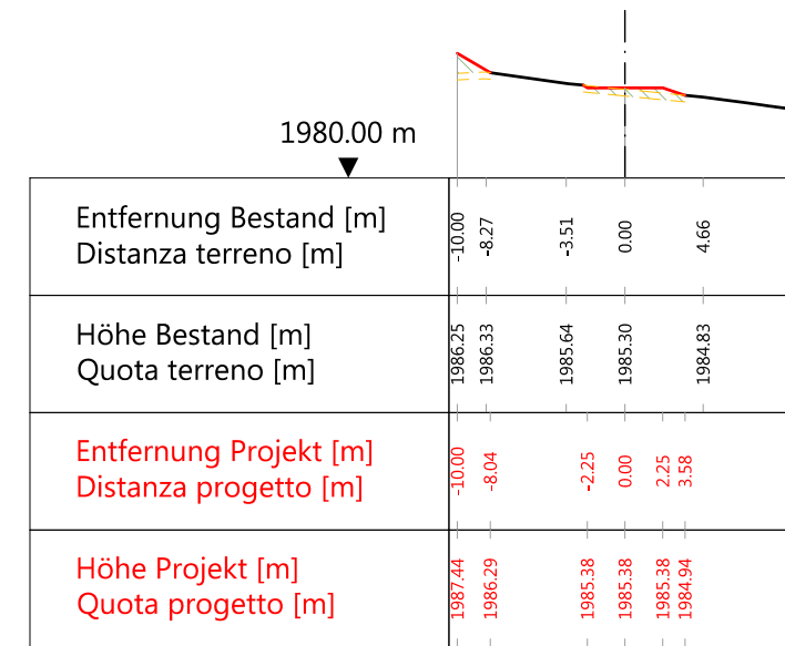
Querprofil L6 Profilo trasversale L6
