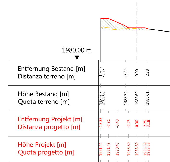
Querprofil L5 Profilo trasversale L5
