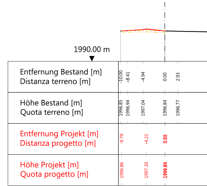
Querprofil L1 Profilo trasversale L1
