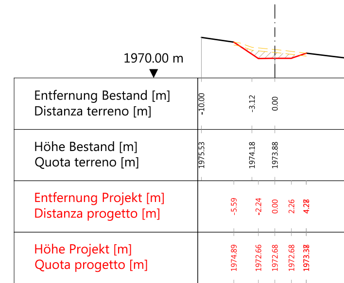
Querprofil L9 Profilo trasversale L9
