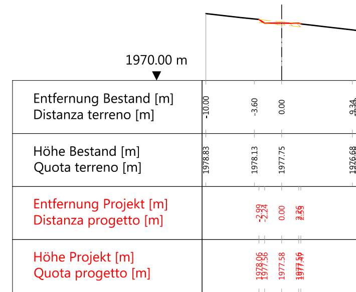
Querprofil L8 Profilo trasversale L8
