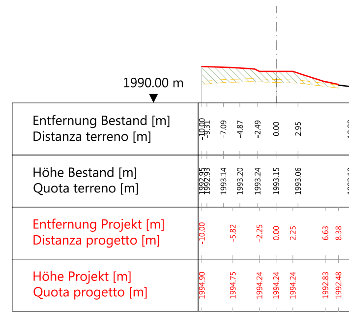
Querprofil L3 Profilo trasversale L3
