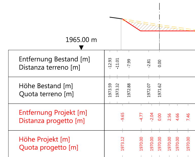
Querprofil L10 Profilo trasversale L10
