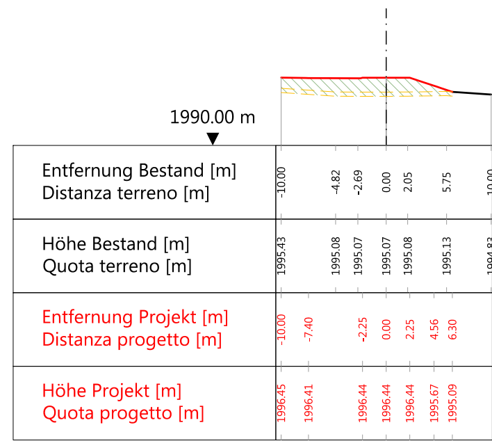
Querprofil L2 Profilo trasversale L2
