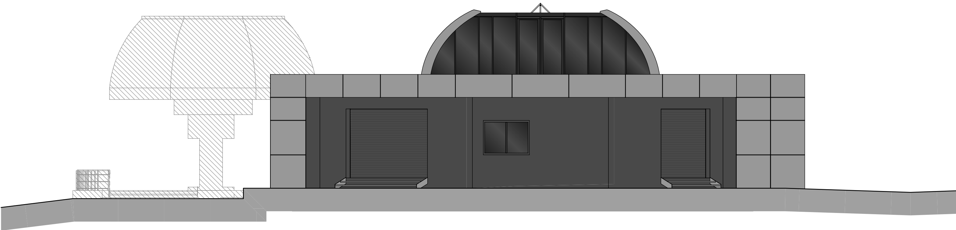
SÜDANSICHT Mst. 1:100
