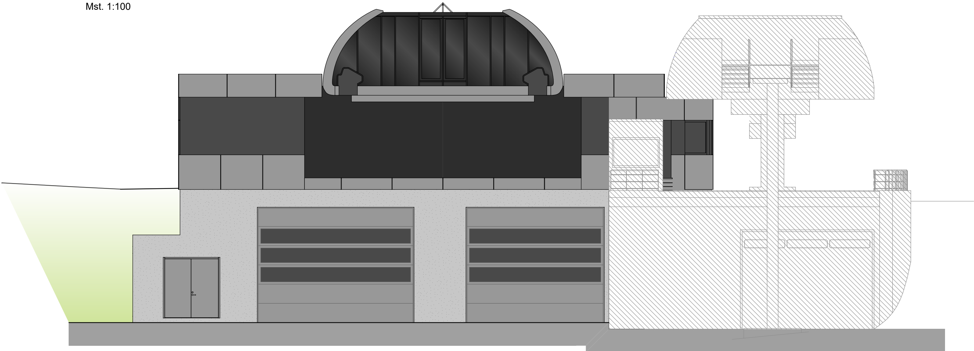
NORDANSICHT Mst. 1:100
