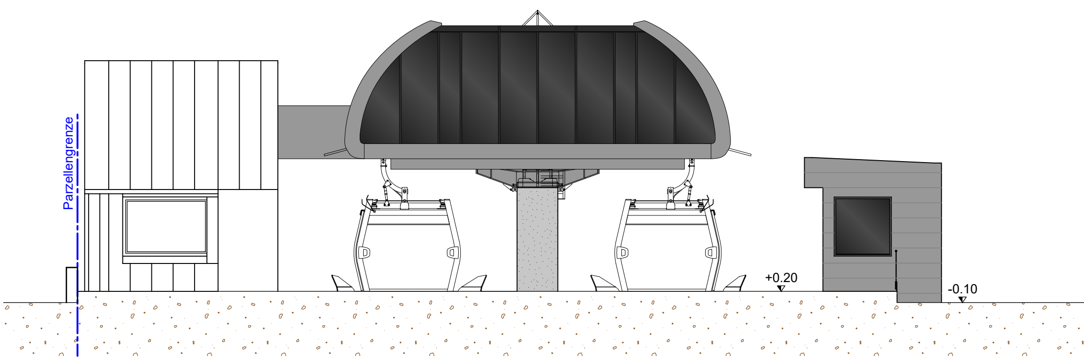
NORDANSICHT Mst. 1:100
