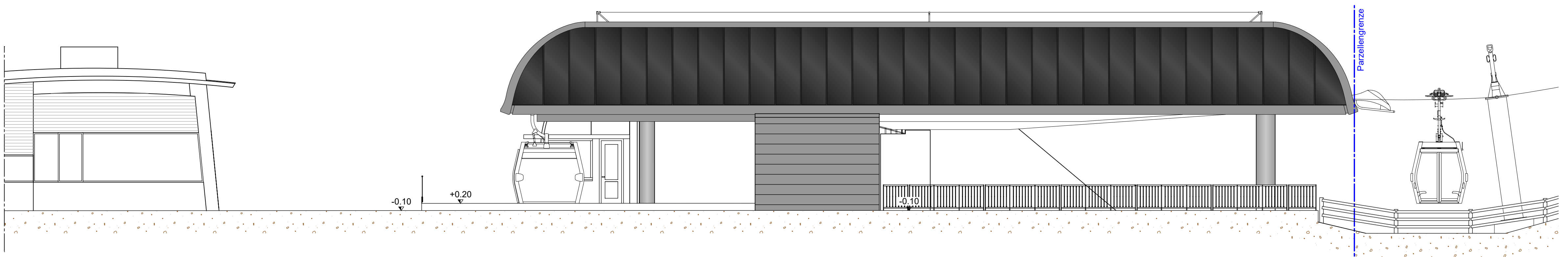
WESTANSICHT Mst. 1:100
