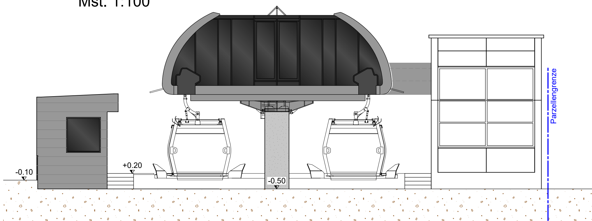
SÜDANSICHT Mst. 1:100
