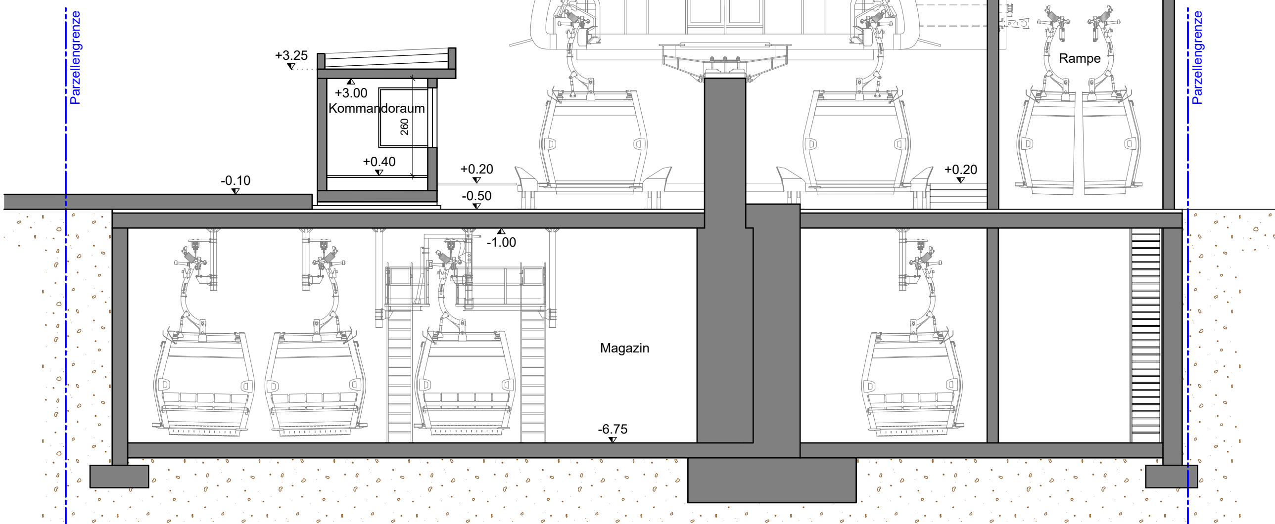
SCHNITT C-C Mst. 1:100
