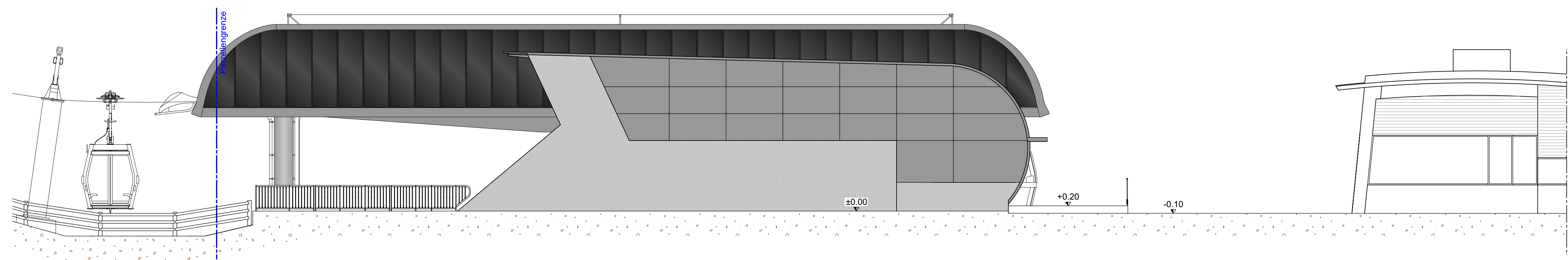
OSTANSICHT Mst. 1:100
