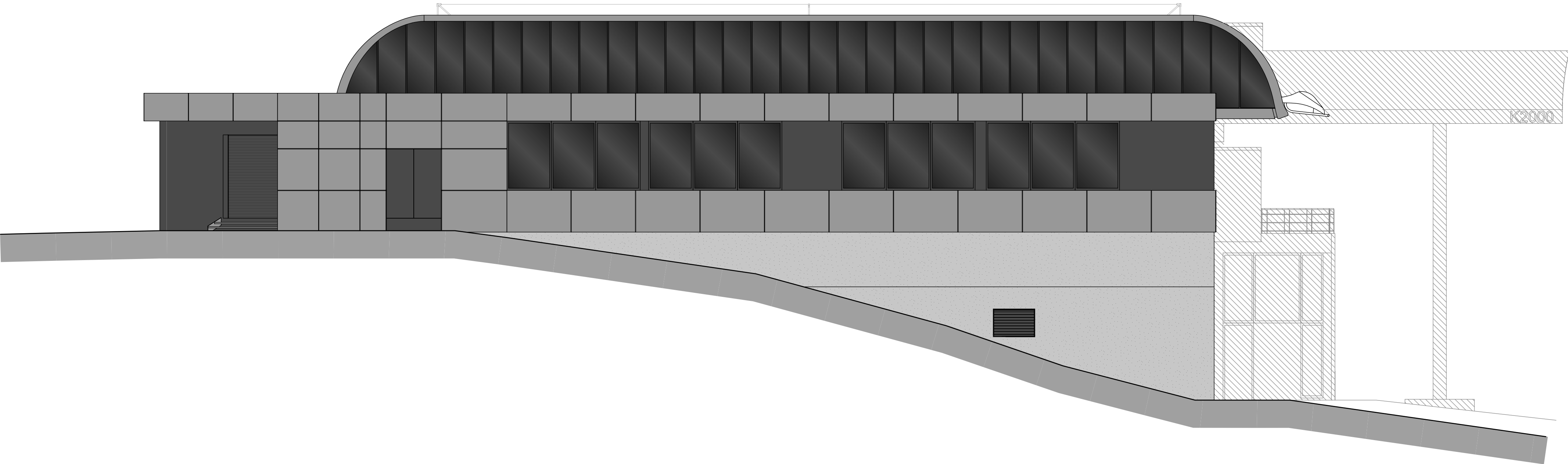
OSTANSICHT Mst. 1:100
