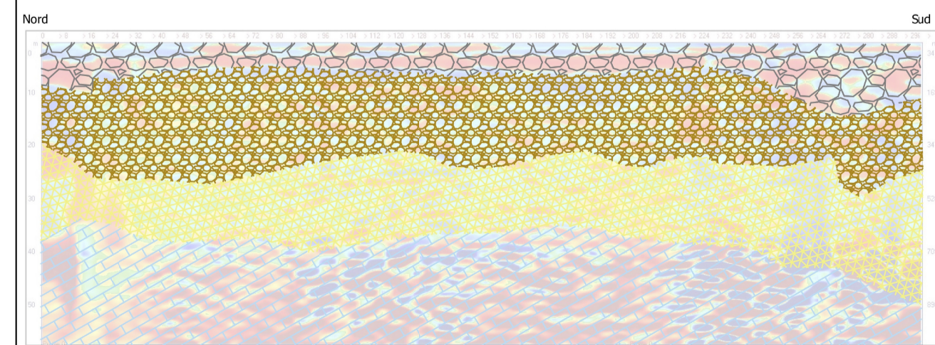
Interpretazione geologica
