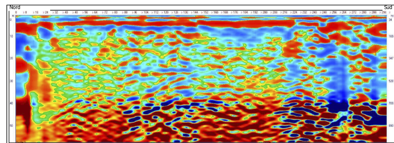
Base Lz1
