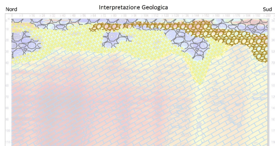
Interpretazione Geologica
