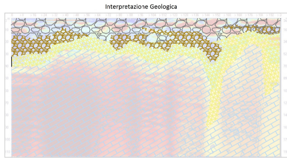
Interpretazione Geologica
