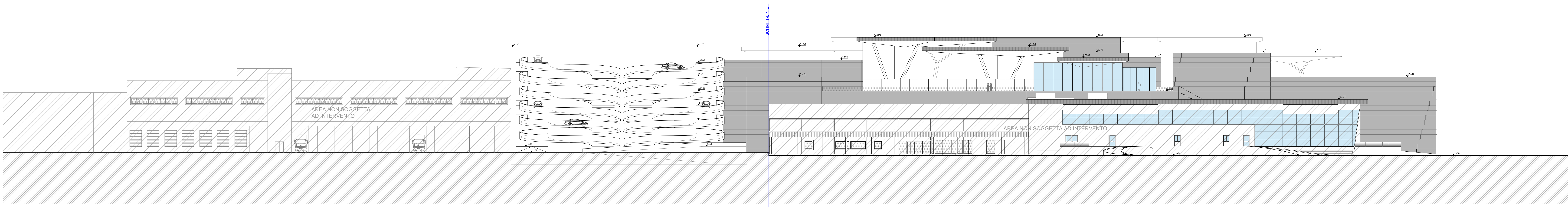
PROSPETTO SUD
