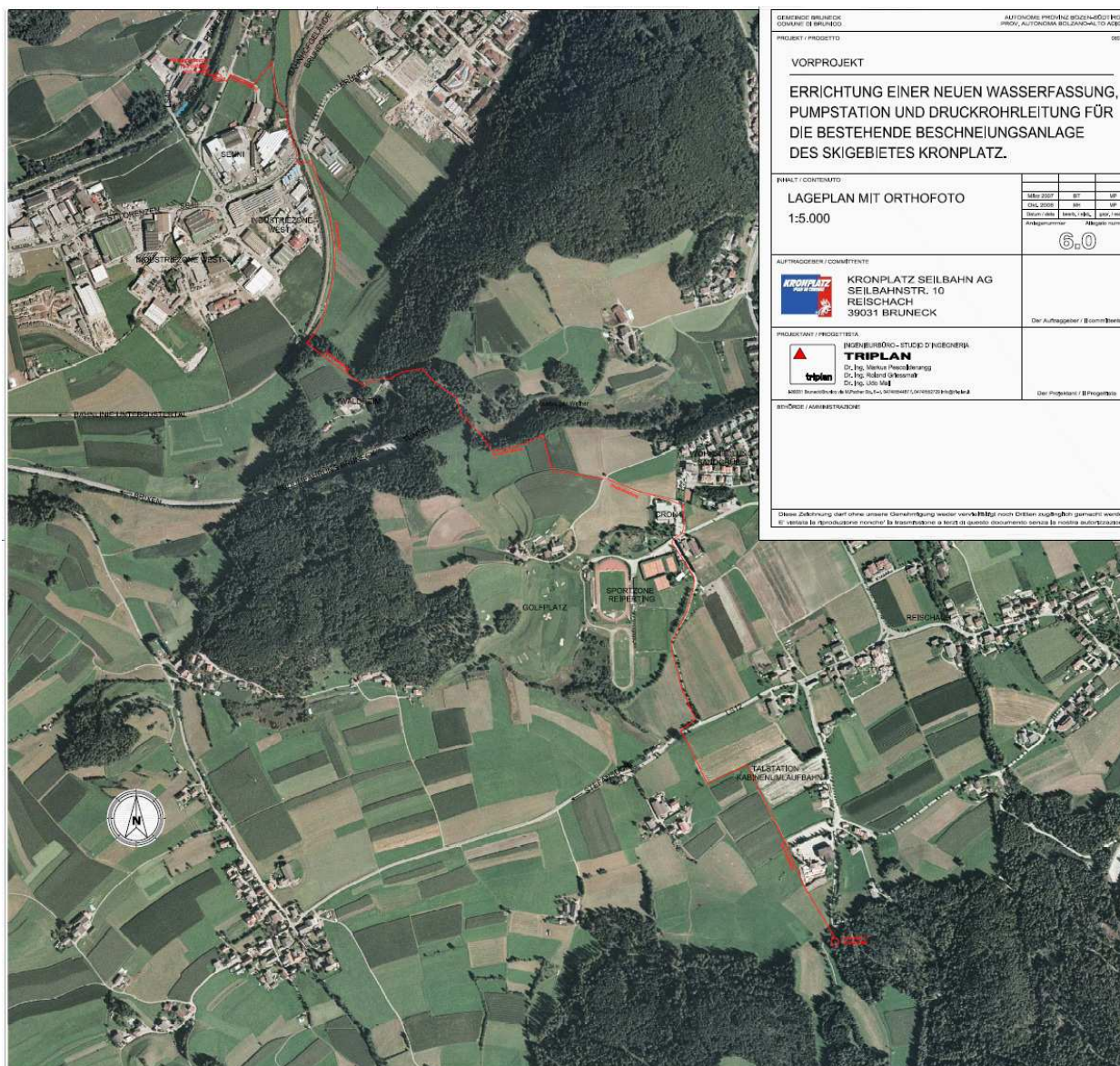
Bild: Orthofoto mit Trassenverlauf der Druckrohrleitung
