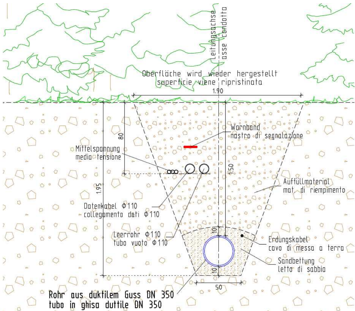
Bild: Regelquerschnitt Druckrohrleitung
