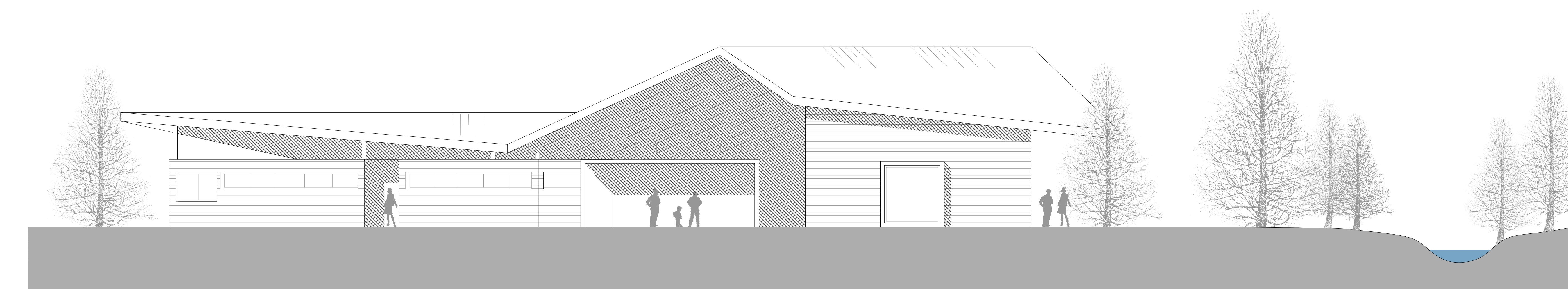
Südwest - Ansicht
