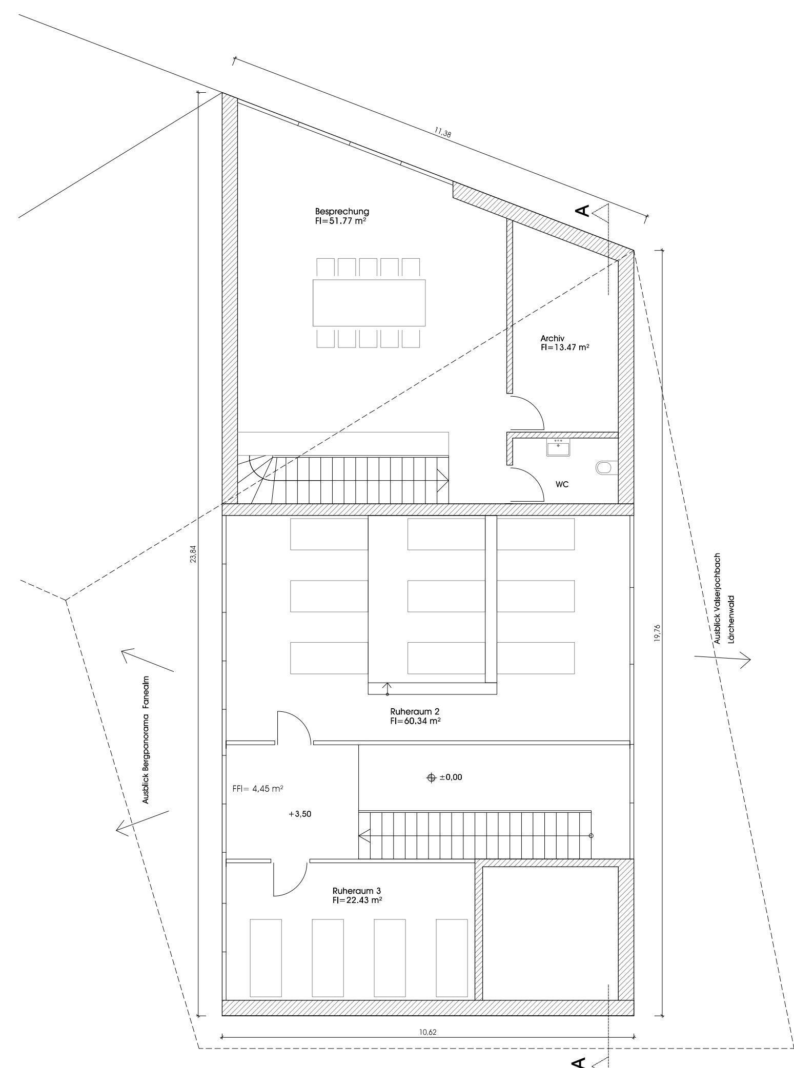
Grundriss Obergeschoss
