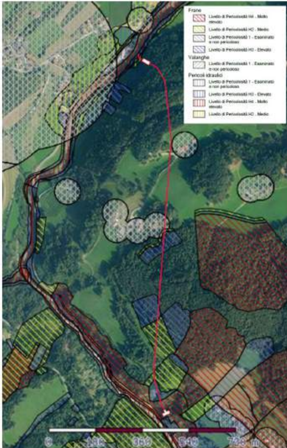
Figura 3-6. Zone di pericolo
