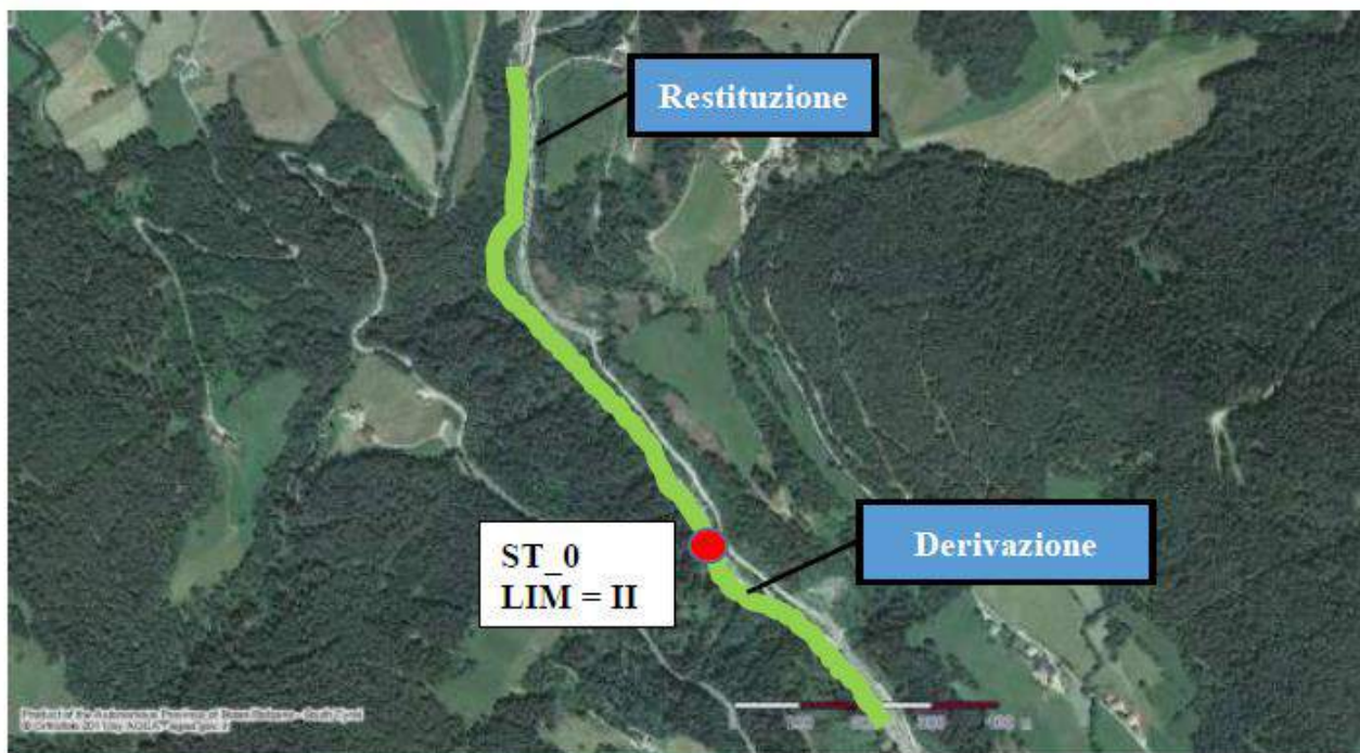
Figura 5-3. Carta di qualità chimico-fisica del rio Gadera espressa dall'indice LIM (ottobre 2014)
