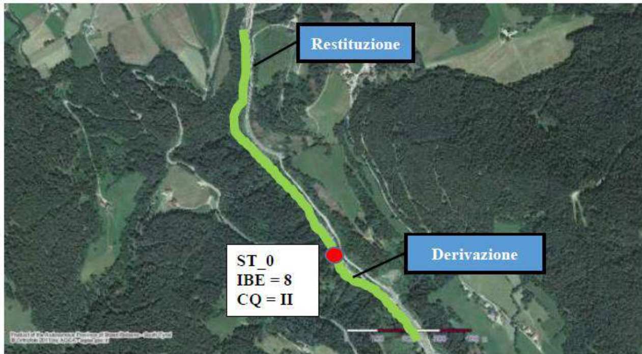
Figura 5-5. Carta di qualità IBE del rio Gadera (ottobre 2014)
