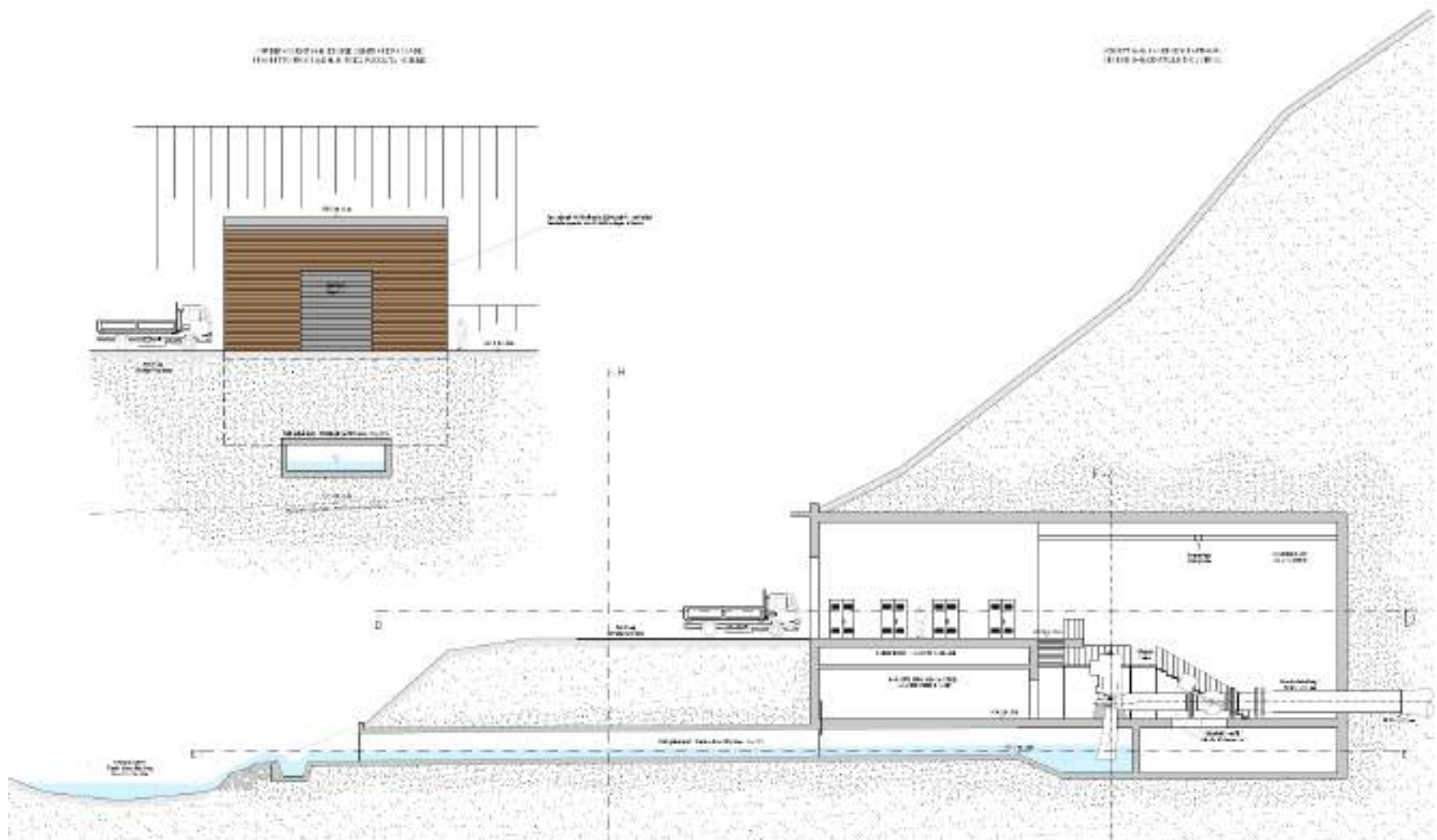
Figura 4-4. Centrale e scarico- prospetto e sezione
