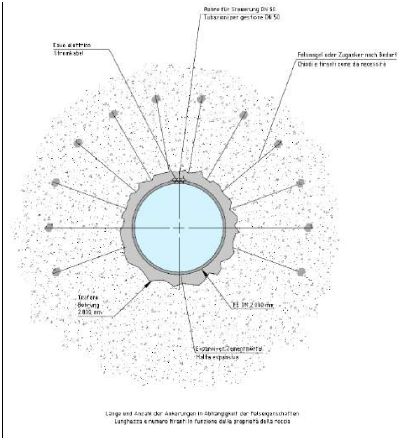
Figura 4-3. Sezione tipo della condotta in galleria
