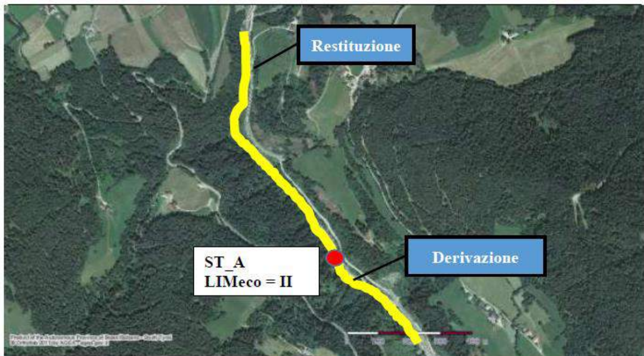
Figura 5-4. Carta di qualità chimico-fisica del rio Gadera espressa dall'indice LIMeco (ott. 2014)
