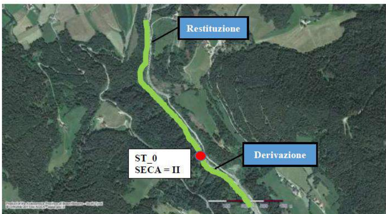
Figura 5-6. Carta di qualità SECA del rio Gadera (ottobre 2014)
