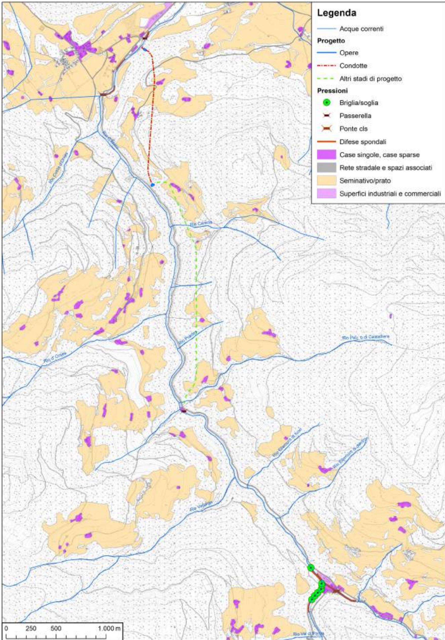
Figura 5-10. Carta delle pressioni
