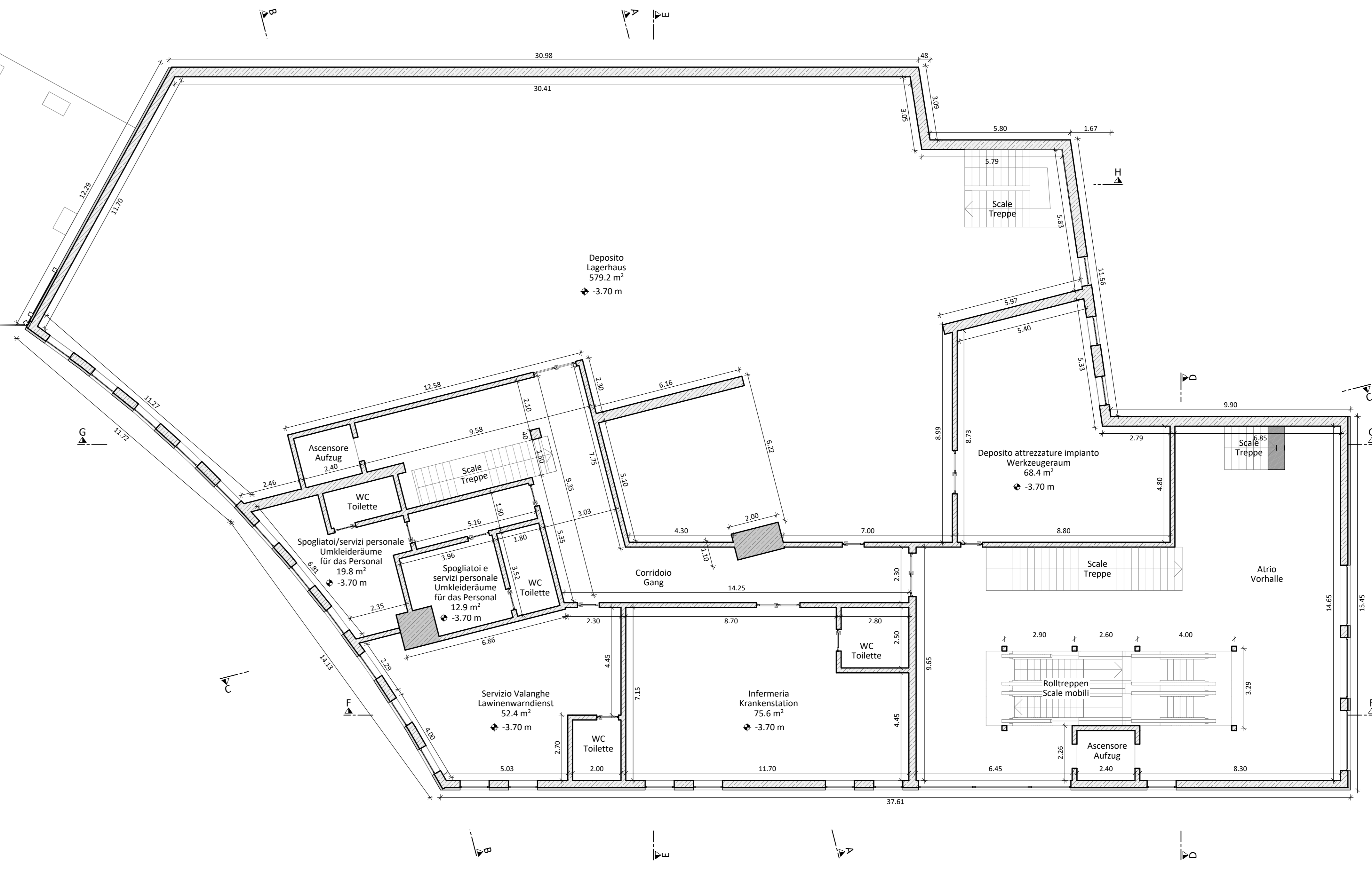
PIANTA PIANO PRIMO M.1:100 GRUDDRISS OBERGESCHOSS QUOTA - HÖHE: -3.70
