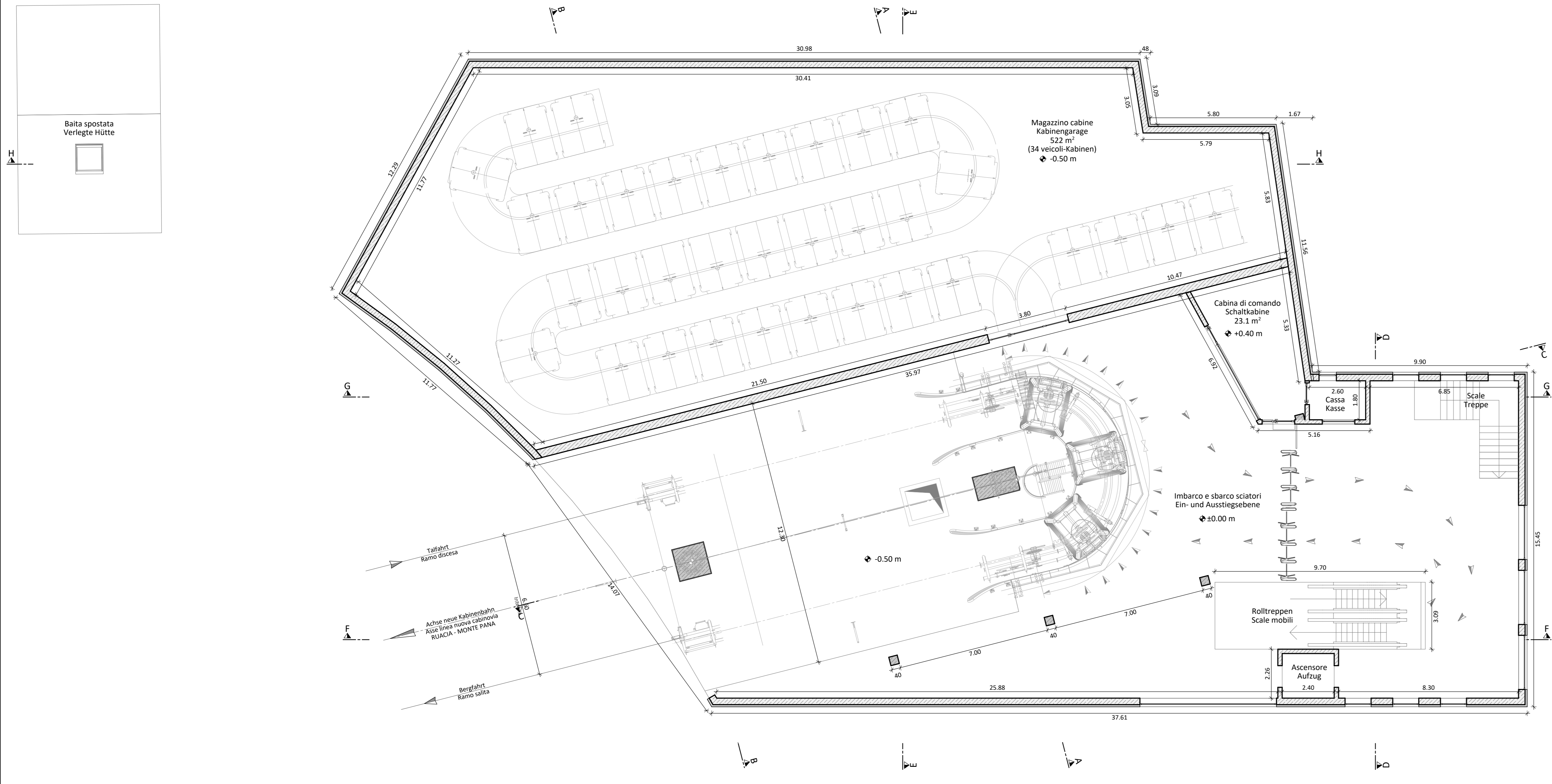
PIANTA PIANO D'IMBARCO E SBARCO M.1:100 GRUDDRISS EIN- UND AUSSTIEGSEBENE QUOTA - HÖHE: ±0.00
