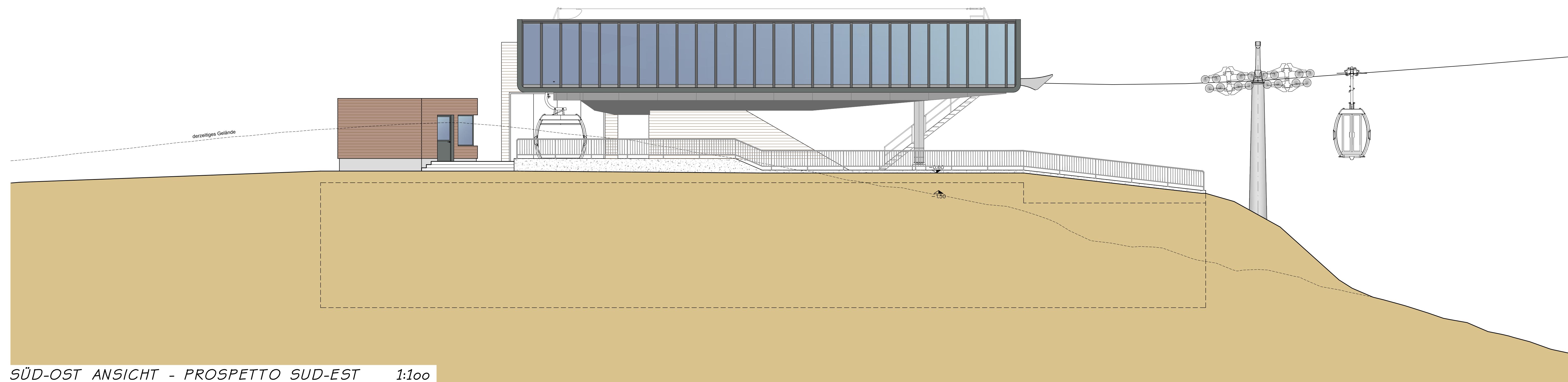
SÜD-OST ANSICHT - PROSPETTO SUD-EST 1:100
