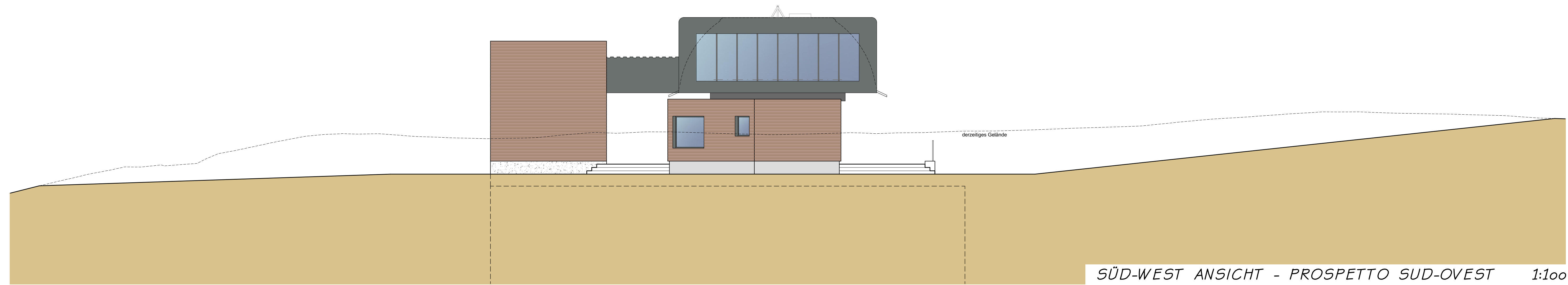
SÜD-WEST ANSICHT - PROSPETTO SUD-OVEST 1:100
