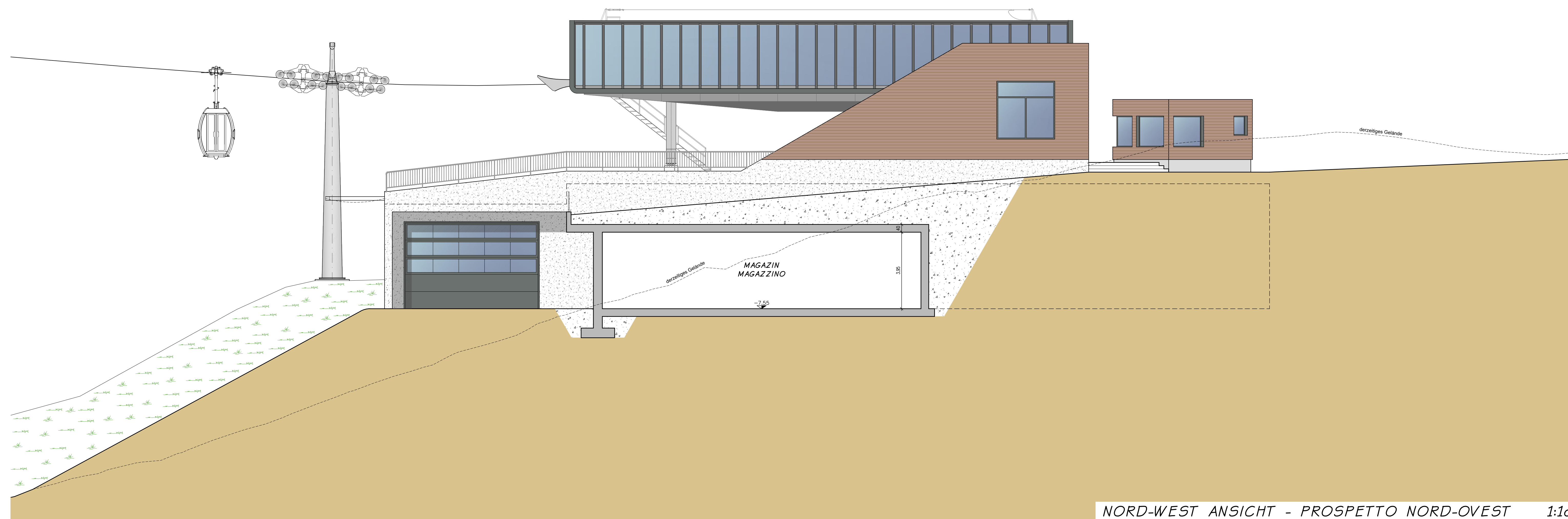
NORD-WEST ANSICHT - PROSPETTO NORD-OVEST 1:100
