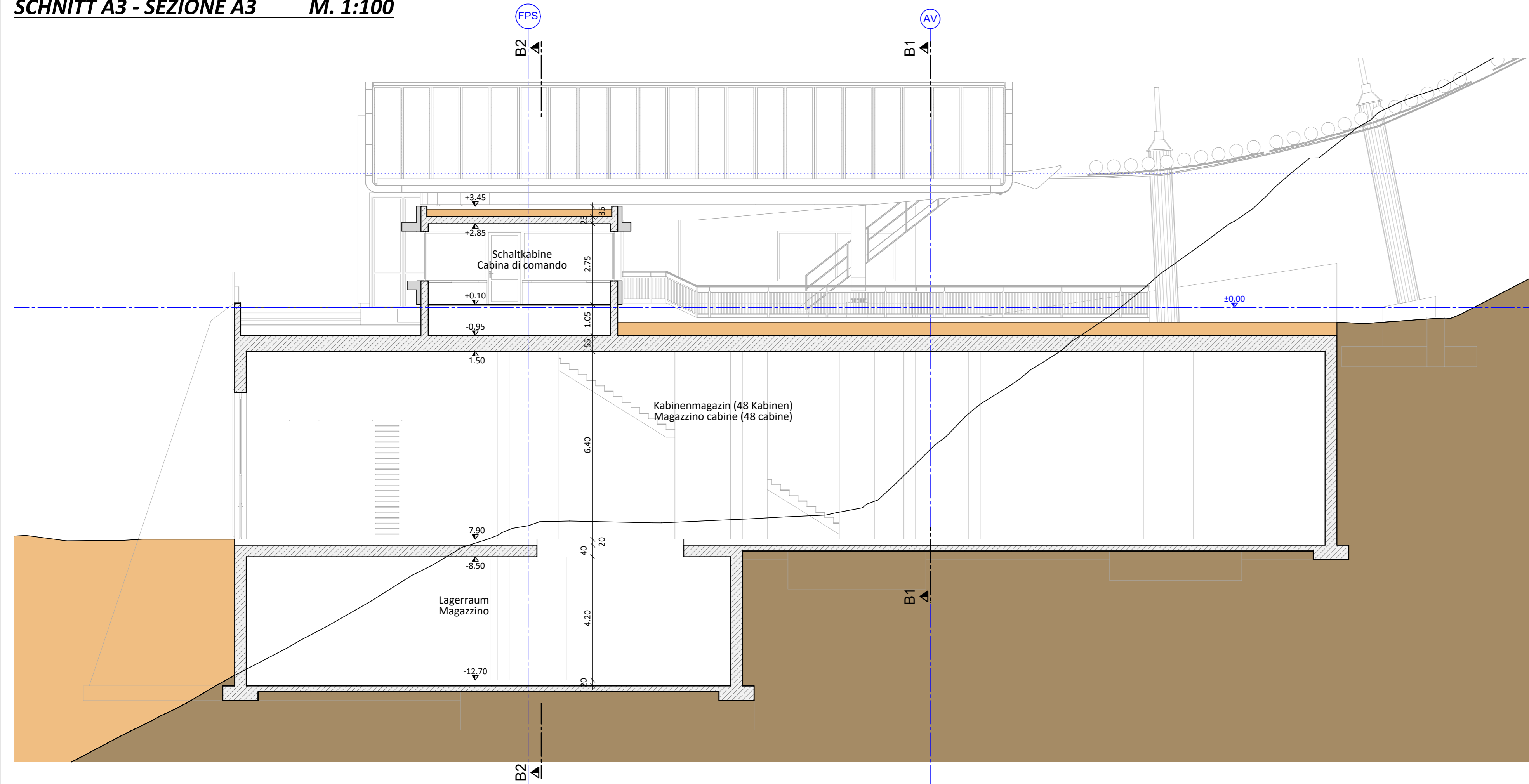
SCHNITT A3 - SEZIONE A3 M. 1:100
