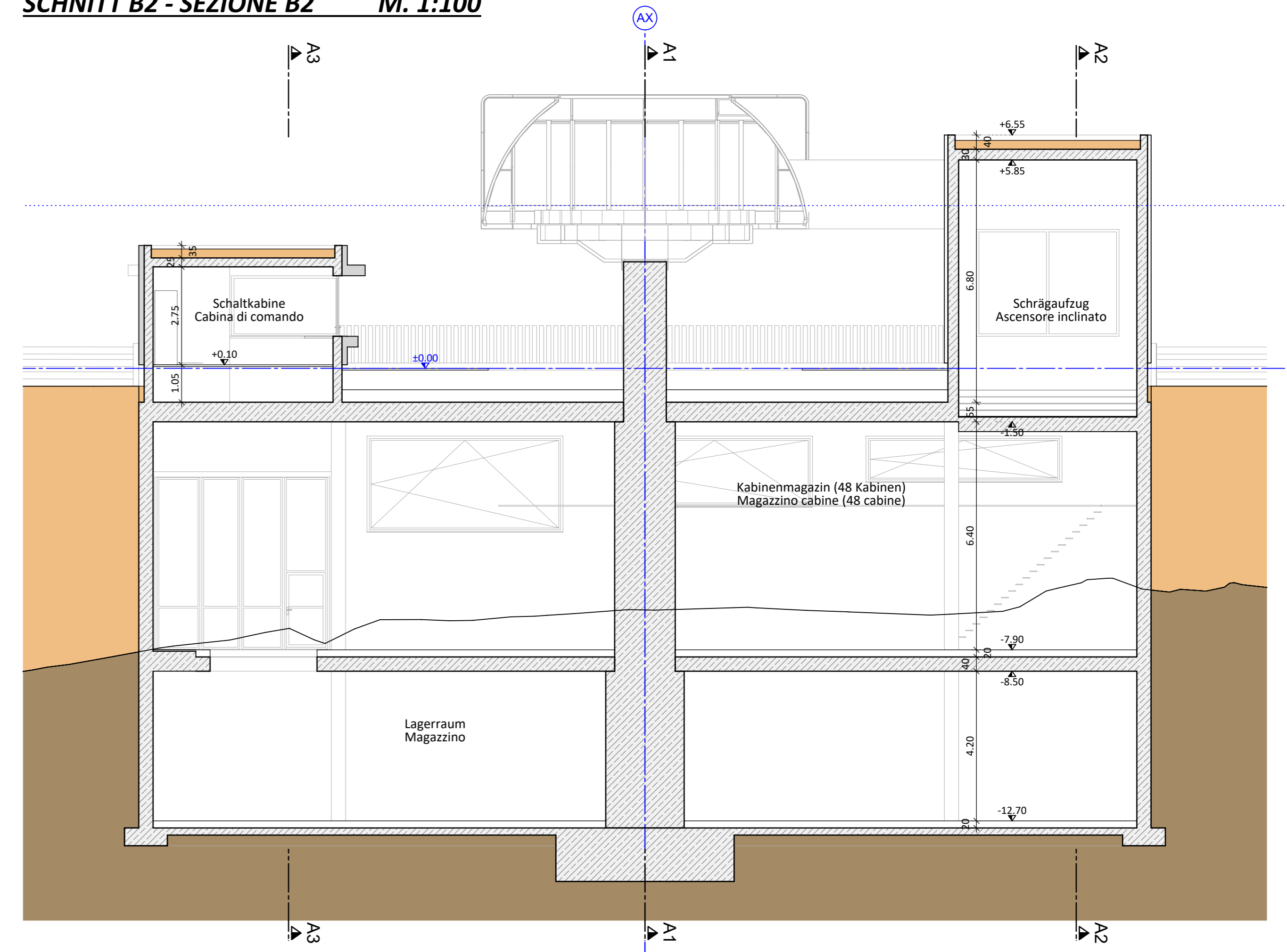
SCHNITT B2 - SEZIONE B2 M. 1:100
