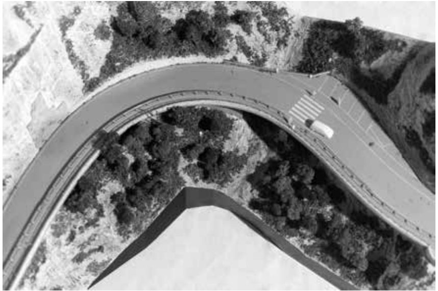
Absicherung der Mendelpasstrasse SS 42 Messa in sicurezza della strada per il passo Mendola SS 42 Rockfall protection tunnel Mendola SS 42
